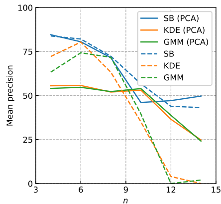
(d) Mean precision vs n
